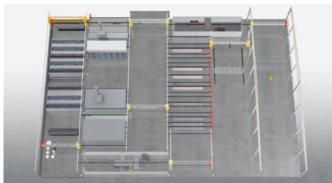
Lackieranlage für Trailer – Gesamtanlage.
