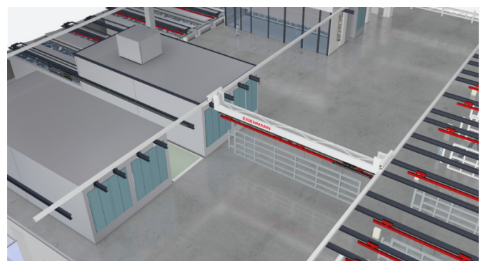
Lackieranlage für Trailer – Transferbrücke mit Wagenzug.
